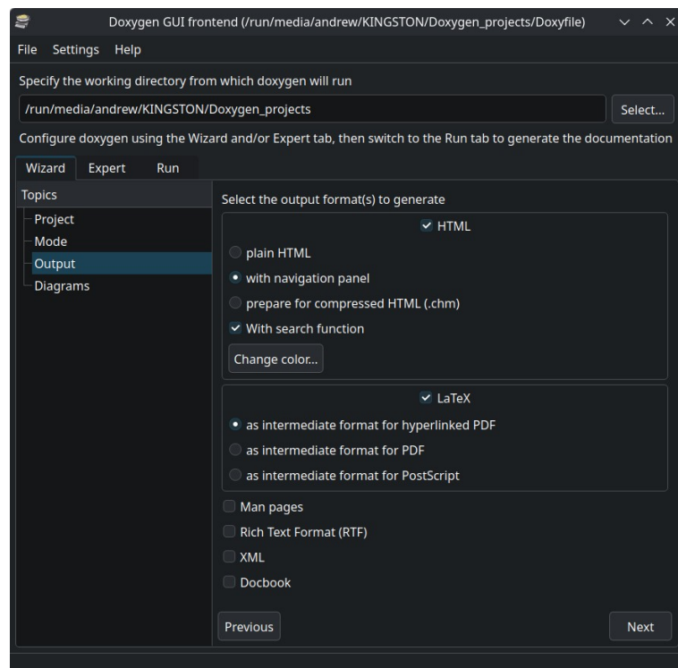
Рисунок 3. Вкладка Wizard -> Output
